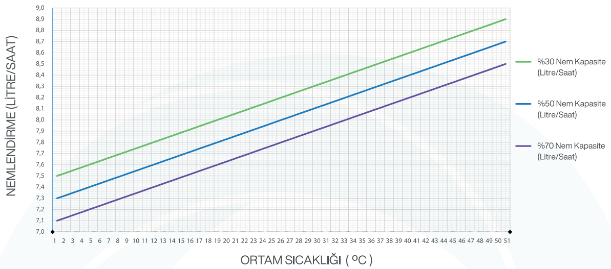
ULTRASONİK NEMLENDİRME CİHAZI TWH-8 KAPASİTE EĞRİSİ
